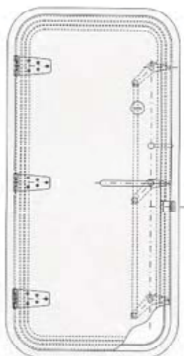
A 型—快开闭风雨密铝质门
