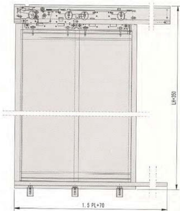
A0电梯旁开双折层门的规格表：
