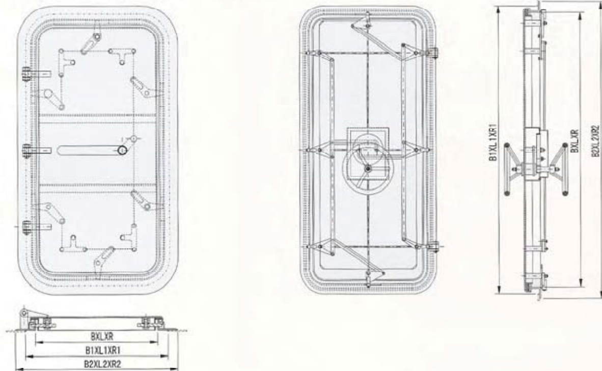
A 型（单把手）
