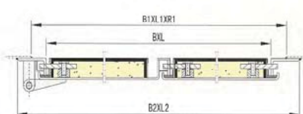
B 型— A60 快开闭风雨密钢质门（双）
