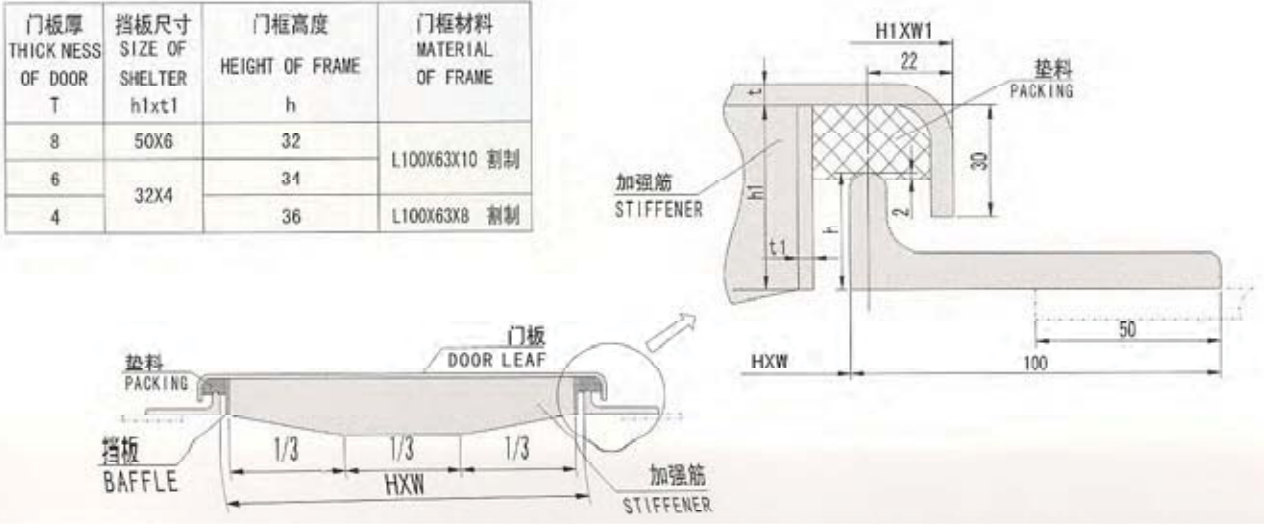
3、门的节点型式 SECTION OF DOOR
