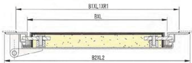
A 型— A60 快开闭风雨密钢质门（单）
